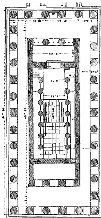
PLAN DU TEMPLE DE ZEUS 1 (PAGE 138).
