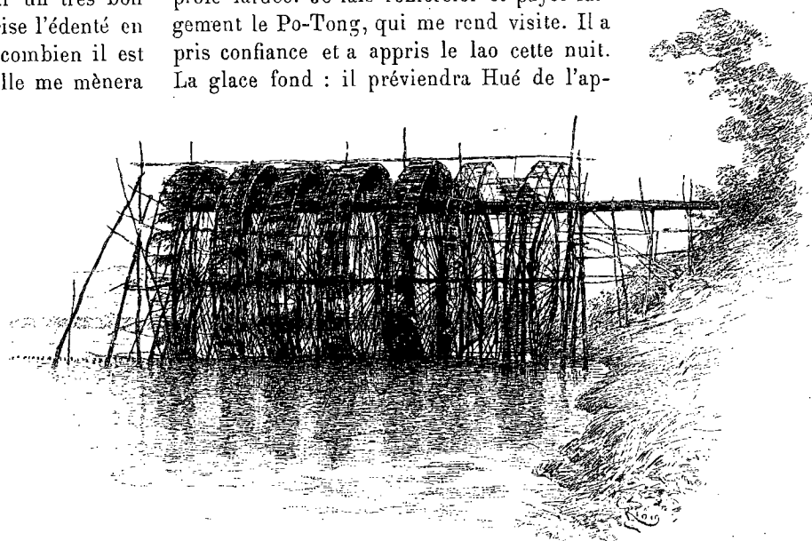
ROUES ÉLEVATRICES 1 (PAGE 388).
