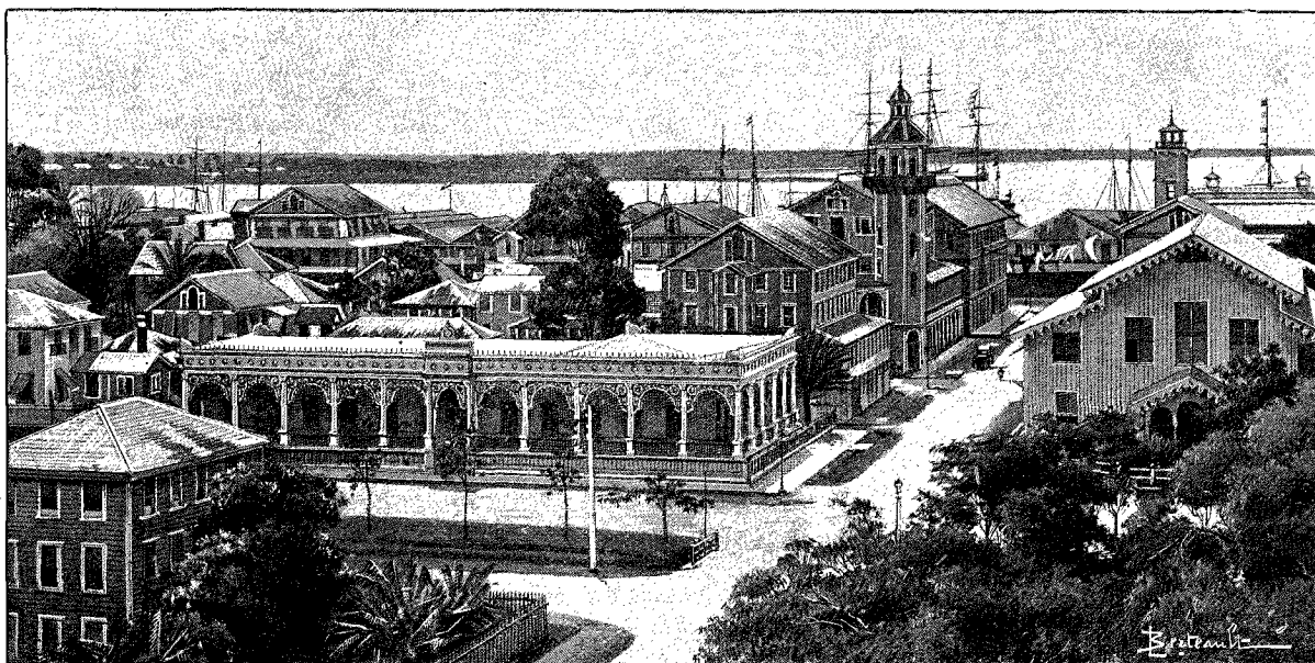
VUE DE GEORGETOWN 1 .
