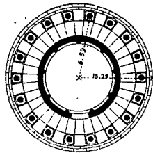
PLAN DU PHILIPPEION 1 .
