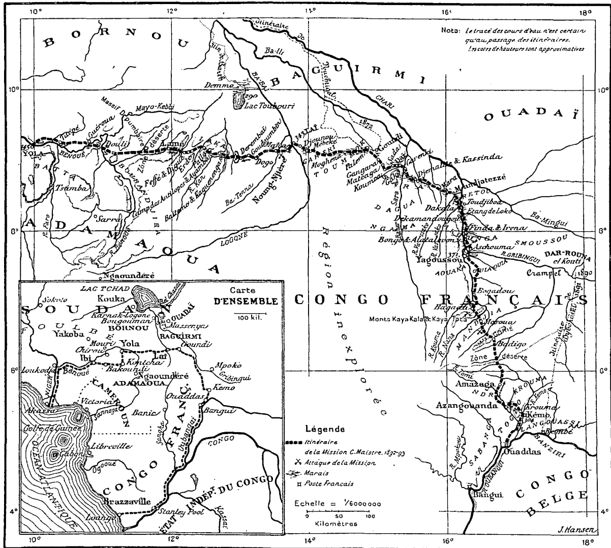
CARTE EXÉCUTÉE D'APRÈS LES DOCUMENTS DE M. C. MAISTRE.
