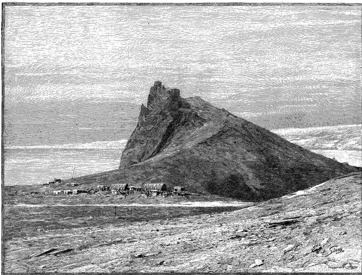
JAN MAYEN : LA STATION AUTRICHIENNE 1 (PAGE 283).
