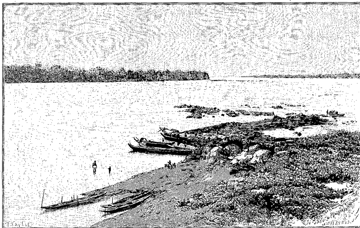
DOUANE SIAMOISE ET RIVIÈRE DE STUNG-TRENG 2 .
