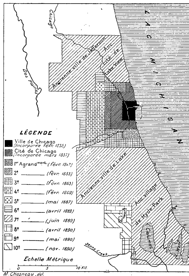
ACCROISSEMENTS SUCCESSIFS DE CHICAGO 1 .
