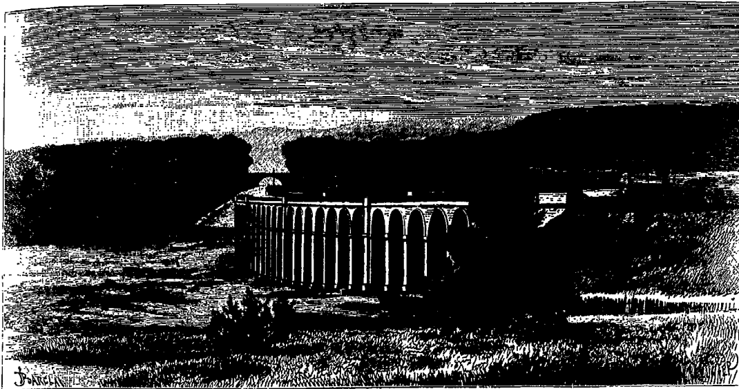
Viaduc du chemin de fer à Dannemarie. — Dessin de Barclay, d'après une photographie.
