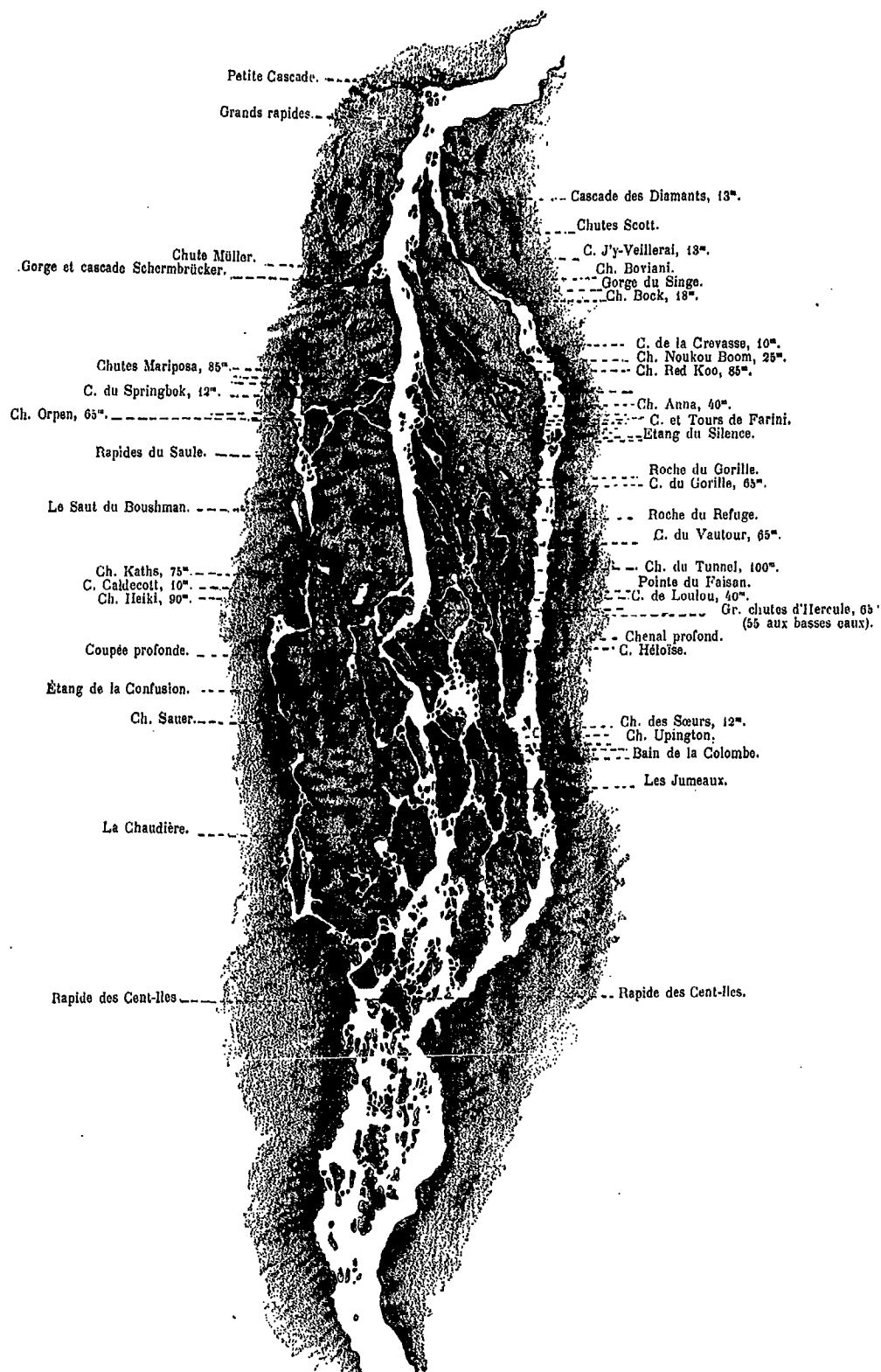
Les rapides et les cascades du fleuve Orange
