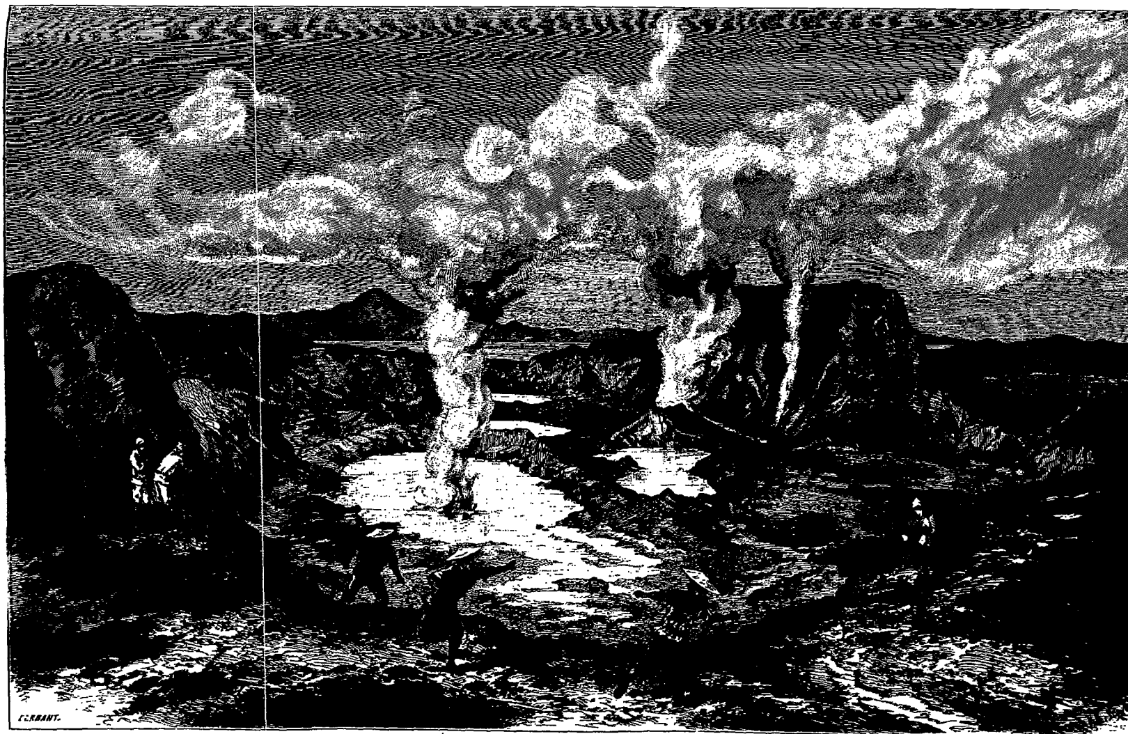
Le volcan Taal (voy. p. 212). — Dessin de Th. Weber, d'après un croquis de M. E. d'Almonde.
