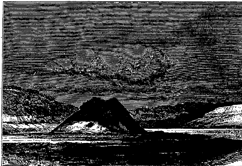
Mont des Singes. — Dessin de Th. Weber, d'après l' Album de Krakatau , publié par le gouvernement hollandais.
