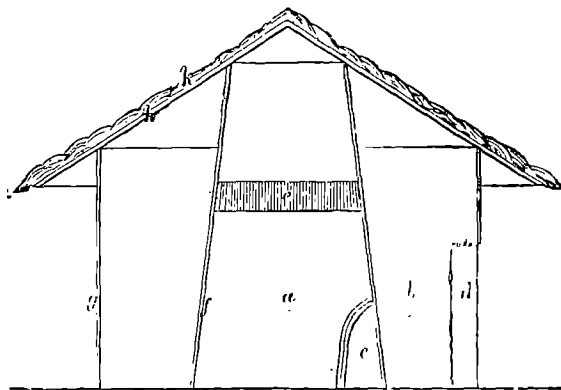
Section verticale d'une maison des Louinas dans le village de Tapa (voy. p. 333).
