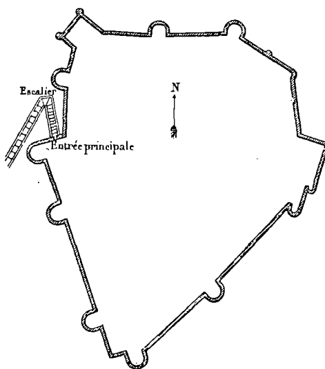
Tibnin Plau de la forteresse (voy. p. 35).
