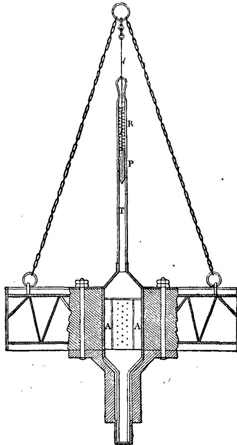
Bouée de sauvetage au phosphore de calcium (coupe) d'après un dessin pris à l'École de pyrotechnie de Toulon.
