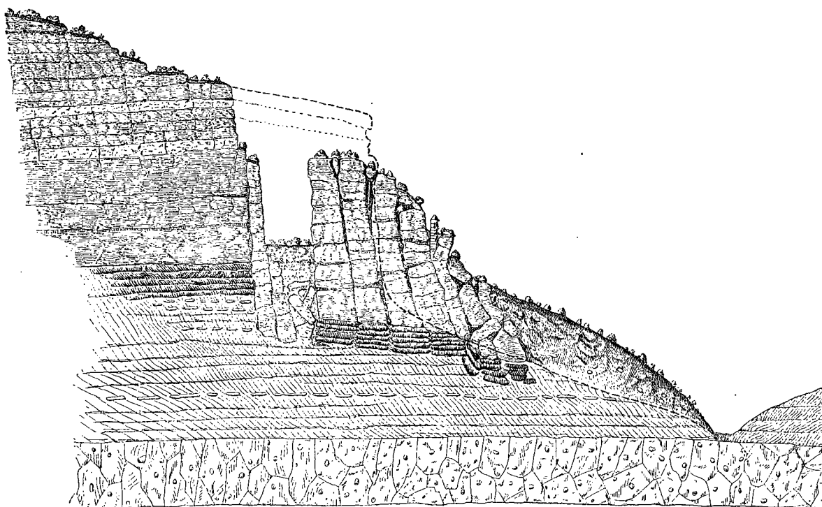
Eboulement de Roquefort (coupe géologique).
