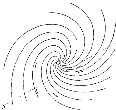
Cyclones.
