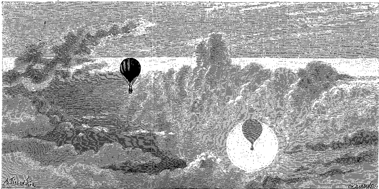
Effet d'ombre aérostatique avec auréole lumineuse, observée au-dessus des nuages, le 19 février 1873. — Dessin d'Albert Tissandier, d'après nature.
