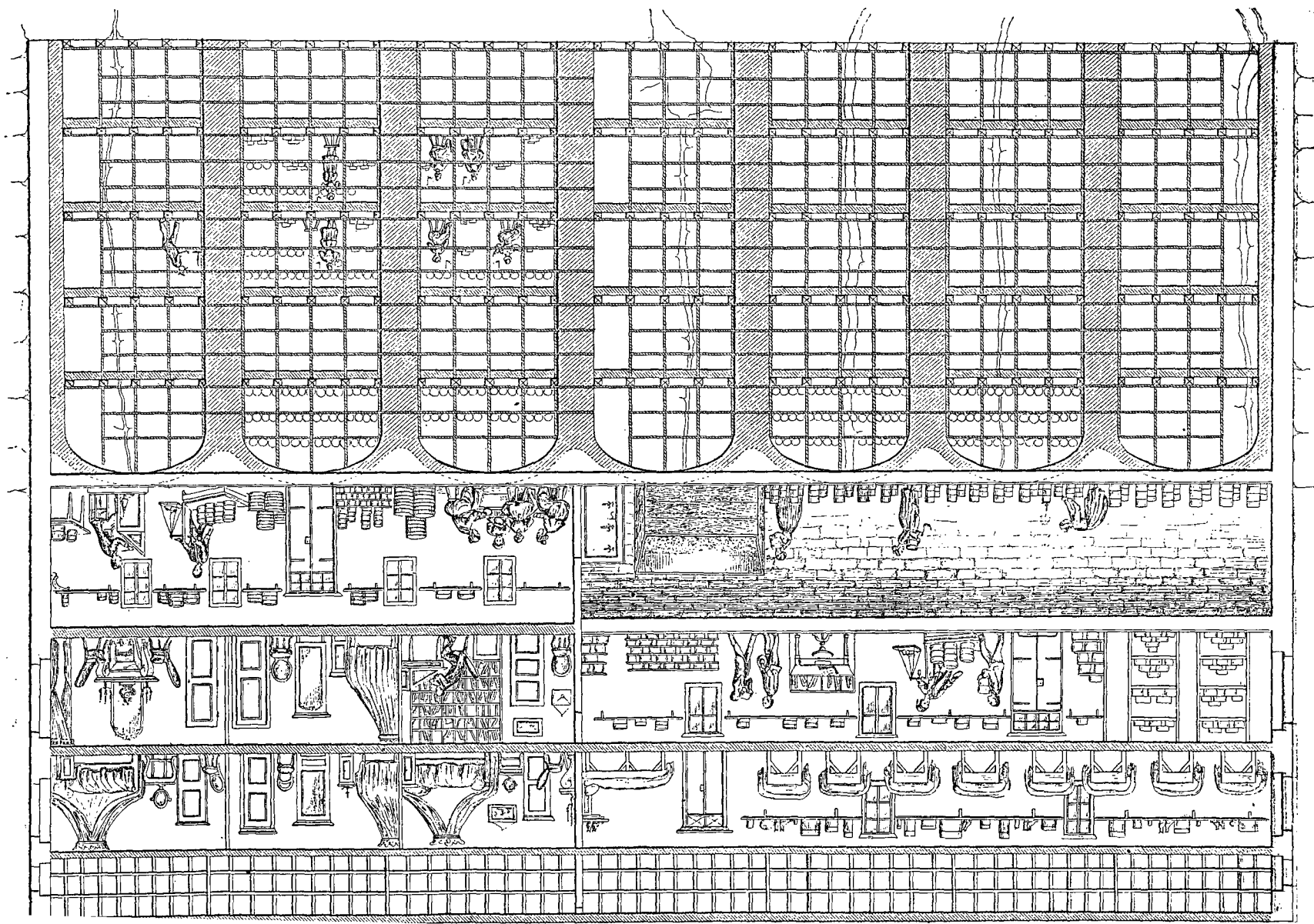
Vue intérieure d'une cave (coupe en long).
