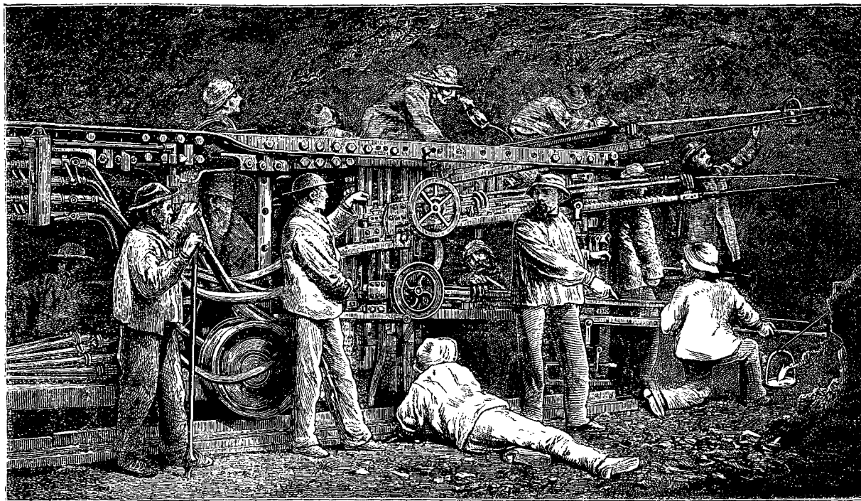
Machine employée au percement du tunnel des Alpes. — Dessin de M. Whympier.
