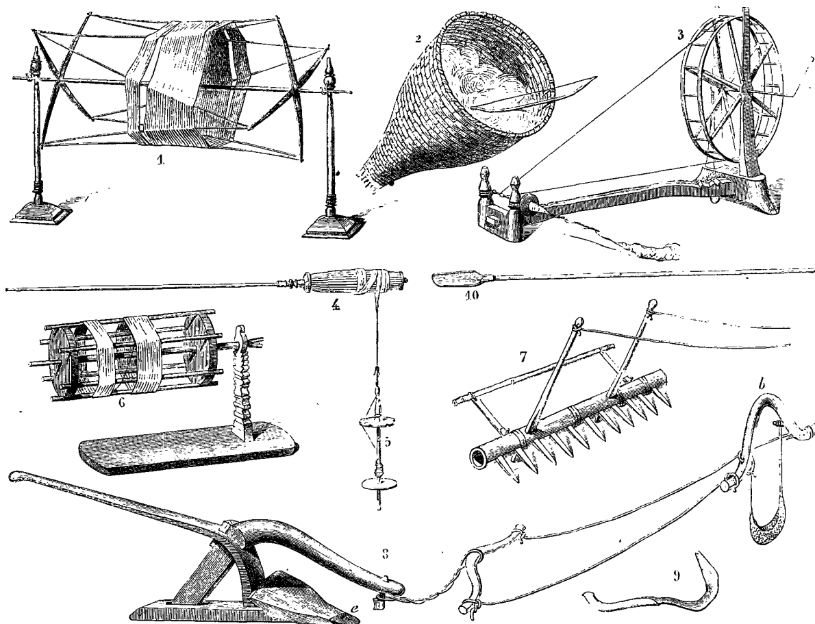
Ustensiles agricoles et textiles au Laos. — Dessin de B. Bonnafoux, d'après un croquis de M. L. Delaporte.
