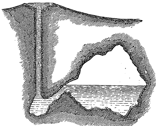
Esquisse théorique du Geiser.
