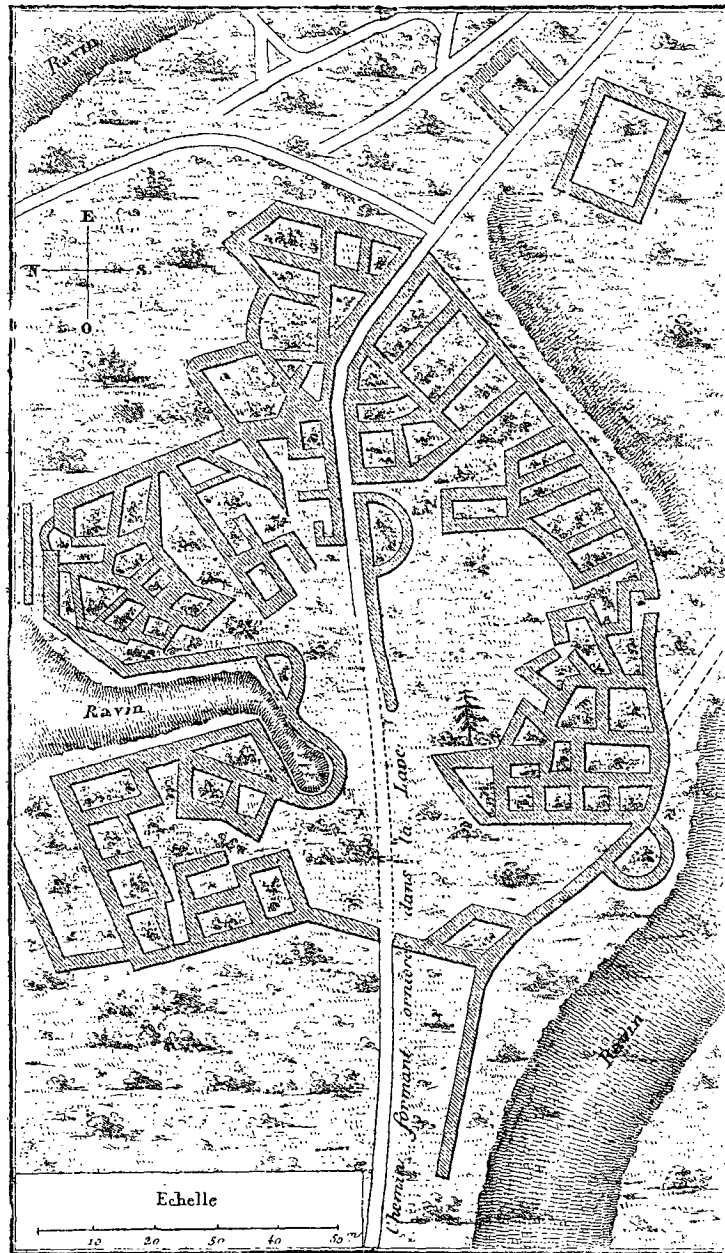
Plan du camp des Chazaloux, ruines gauloises près de Pontgibaud.
