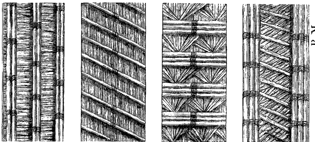
Appareils de toiture en usage dans la pampa del Sacramento.
