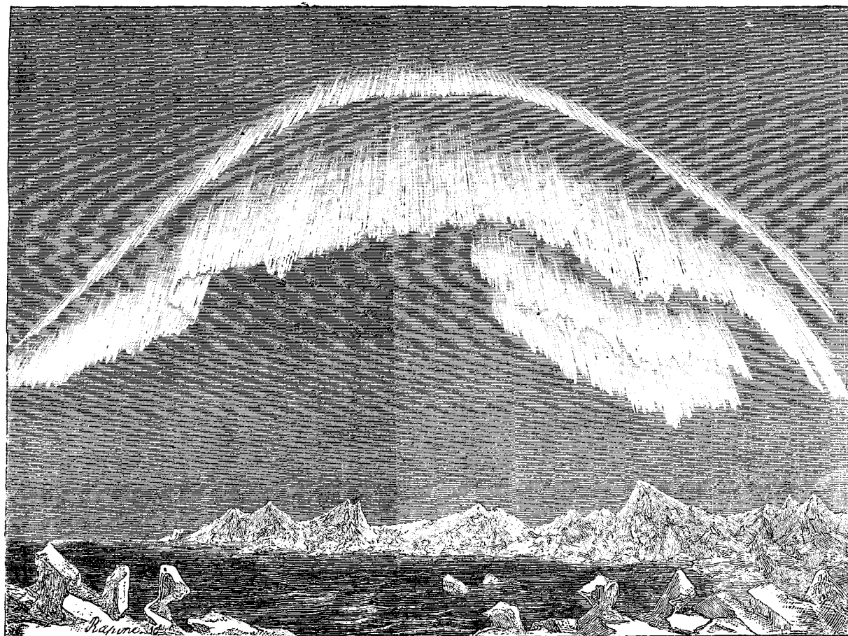
Apparence de l'aurore boréale dans le nord, à Bossekop (Finmark) le 6 janvier 1839, à 6 h. 27 min. du soir. Dessin et gravure de Rapine d'après Bévalet.
