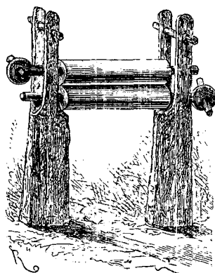
Moulin à broyer les cannes à sucre.
