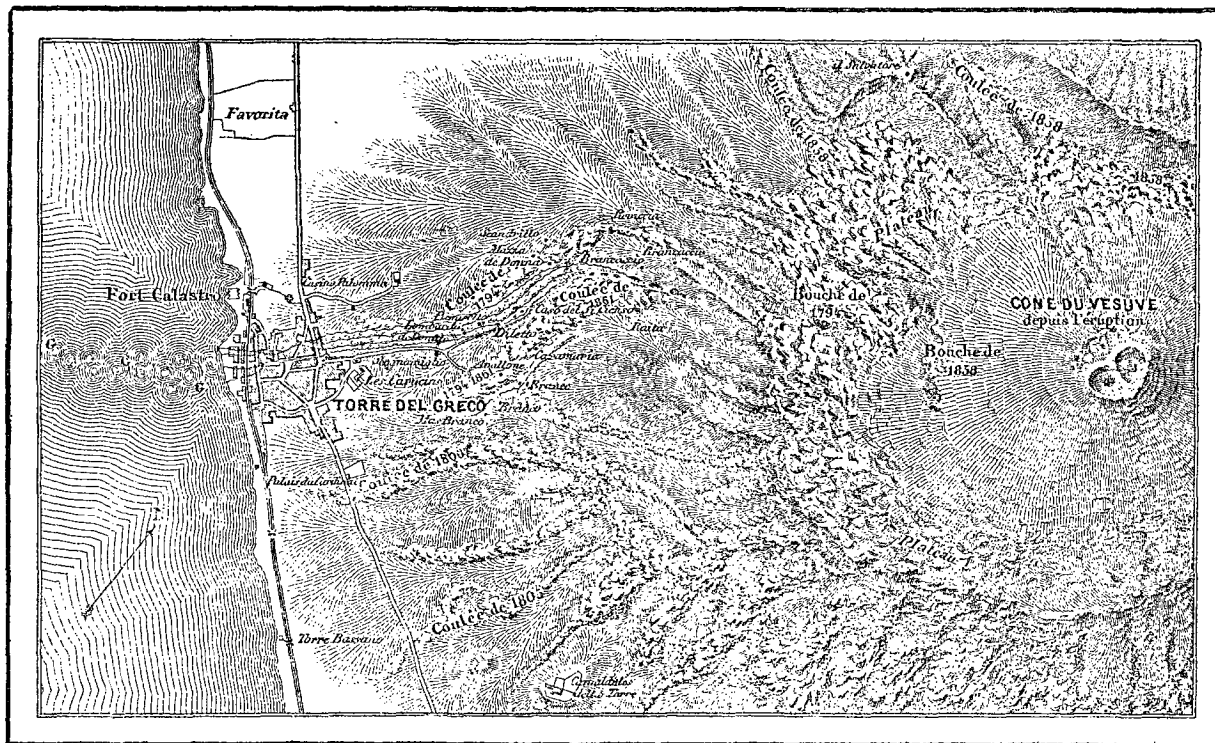
Gravé chez Erhard, R. Bonaparte 42. Carte de la région du Vésuve bouleversée par les phénomènes volcaniques de décembre 1861 à février 1862. G, G, G. Bouillonnements de la mer le 8 décembre 1860.
